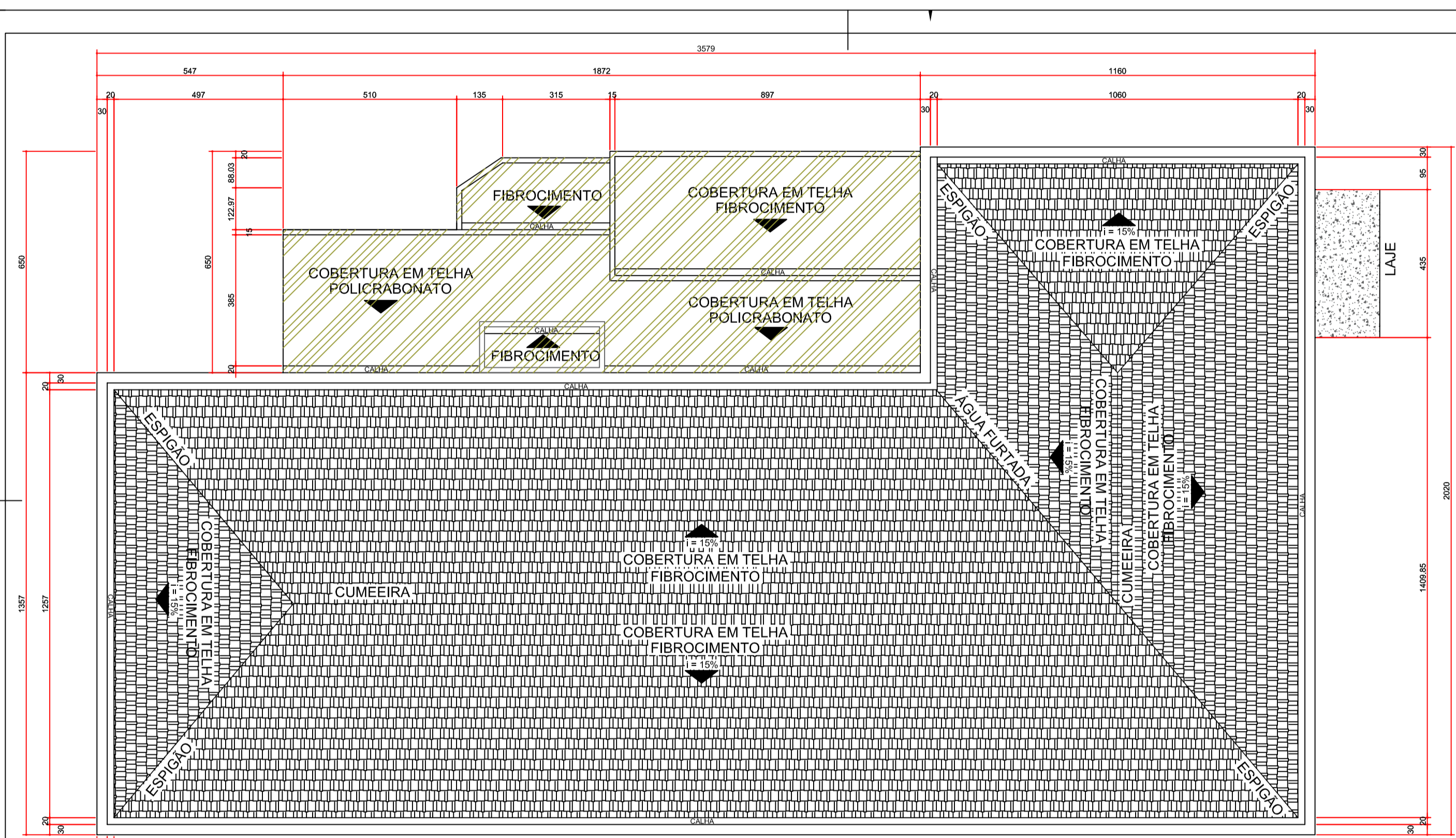
PLANTA TELHADO ESCALA 1:100
